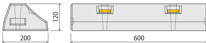
パーキングブロックⅡ (穴あき, 反射板付, H120)
