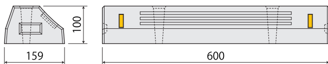
パーキングブロックⅣ (穴あき, 反射板付, H100)
