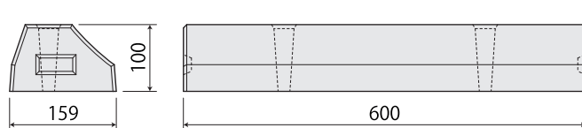
パーキングブロックⅢ (穴あき, H100)
