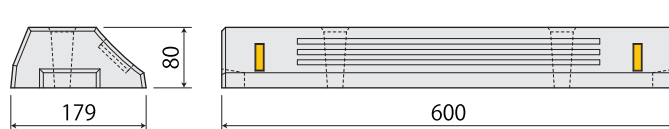
パーキングブロックⅤ (穴あき, 反射板付, H80)
