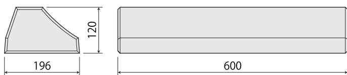
パーキングブロック 標準 H120
