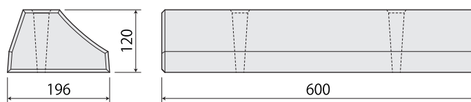
パーキングブロック 穴あき H120
