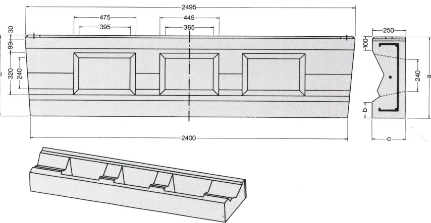
■寸法表 (3分勾配)
